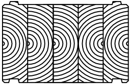
Lamellihiri 330 x 205 Kuusi ja mänty
