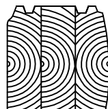
Lamellihiri 200 x 205 Kuusi ja mänty
