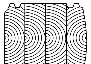
Lamellihirsi 270 x 205 Kuusi ja mänty
