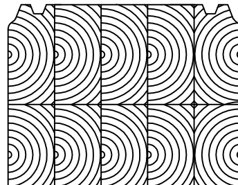
Lamellihirsi 330 x 270 Kuusi
