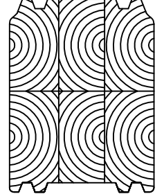
Lamellihirsi 205 x 260 Kuusi
