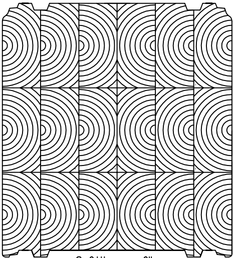
Lamellihirsi 450 x 485 Kuusi
