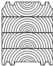
Lamellihirsi 212 x 250 Kuusi
