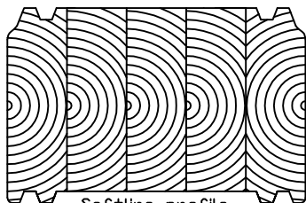
Lamellihirsi 330 x 203 Kuusi ja mänty
