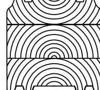
Lamellihirsi 190 x 183 Kuusi
