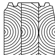
Lamellihirsi 200 x 205 Kuusi ja mänty
