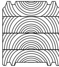
Lamellihirsi 235 x 250 Kuusi
