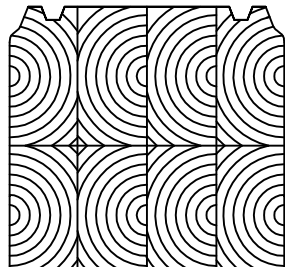
Lamellihirsi 270 x 260 Kuusi
