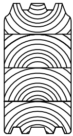
Lamellihirsi 135 x 250 Kuusi
