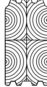
Lamellihirsi 135 x 260 Kuusi
