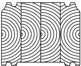
Lamellihirsi 270 x 203 Kuusi ja mänty
