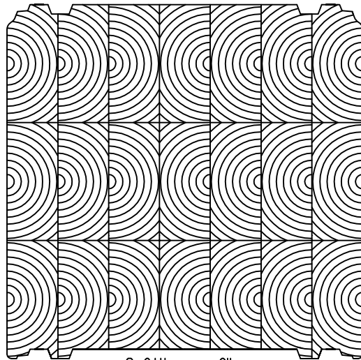
Lamellihirsi 500 x 485 Kuusi
